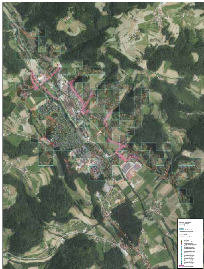
Pregledna situacija za sekundarno kanalizacijo
