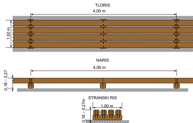
NAČRTOVANA POT – VARIANTA 1
